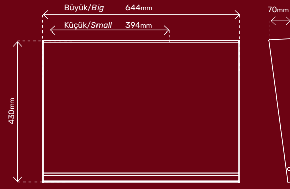
Küçük Sebze ve Köfte Pişirici Small Vegetable and Meatball Cooker
